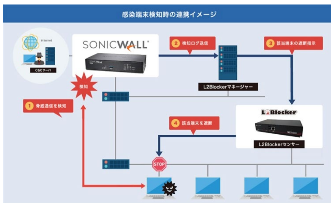
L2Blocker と SonicWall 次世代ファイアウォール の連携イメージ
